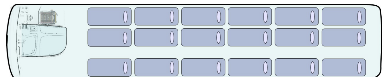
TF25 13.5 G6R - 36 (2x1) Sleeper berth with FOH door
